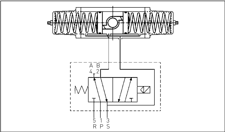
Einfach wirkend mit Namur 5/2-Weg-Ventil
