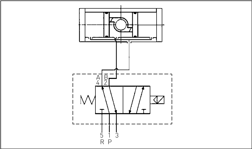
Doppelt wirkend mit Namur 5/2-Weg-Ventil
