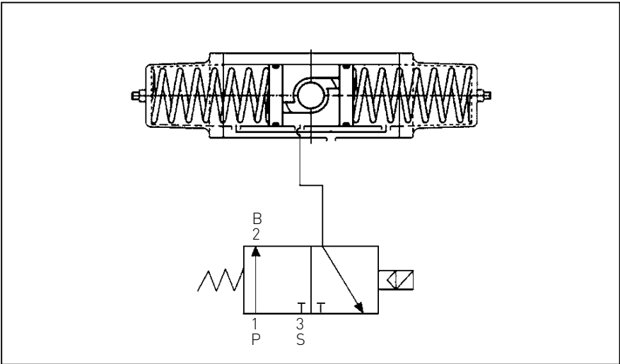
Einfach wirkend mit 3/2-Weg-Ventil
